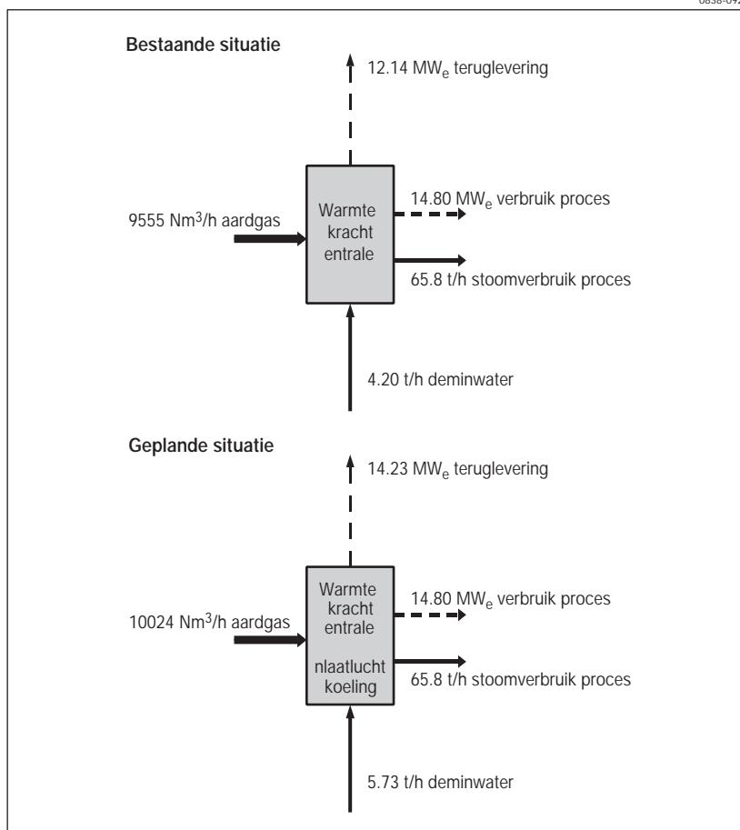
Figuur 8. Energiestromen warmtekrachtcentrale met en zonder modificatie.
