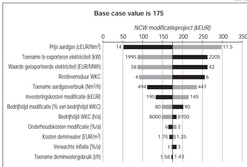
Figuur 10. Tornado diagram gevoeligheden modificatieproject. Dit tornado diagram werd gemaakt met een voor Excel geschreven macro, die onder andere de bar chart gebruikt. Er zijn ook commerciële programma's die hetzelfde voor u doen 1 .
